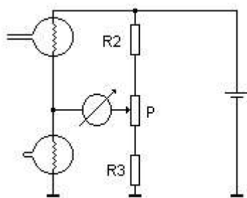
Rys.2 Układ próżniomierza z kompensacją
