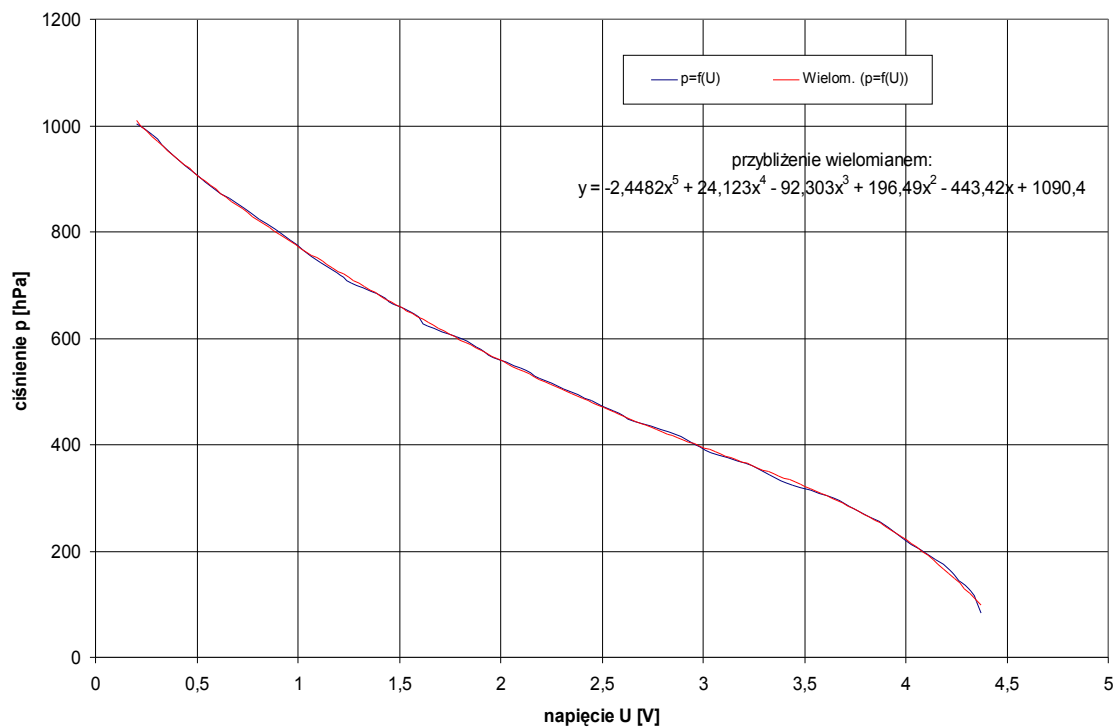
Rys.6. Ciśnienie jako funkcja napięcia na wyjściu wzmacniacza operacyjnego i aproksymacja tej funkcji wielomianem piątego stopnia. Napięcie żarzenia czujnika U_{\text{ż}}=0,45 , ciśnienie atmosferyczne p_{\text{atm}}=753\text{mmHg} , wilgotność względna 50%
