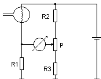
Rys. 1. Zasada działania próżniomierza Piraniego
