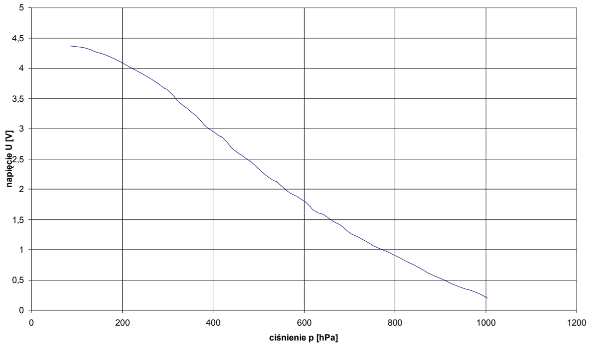
Rys.5.Przebieg napięcia na wyjściu wzmacniacza operacyjnego jako funkcja ciśnienia powietrza dla czujnika pracującego w modelu wykonanym przez autora. Napięcie żarzenia czujnika U_z=0,45V , ciśnienie atmosferyczne p_{atm}=753mmHg , wilgotność względna 50%
