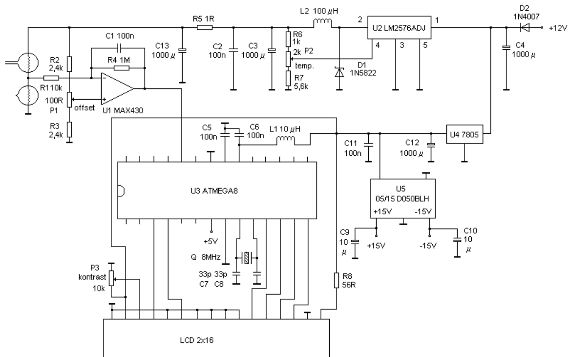
Rys. 3 Schemat elektryczny próżniomierza
