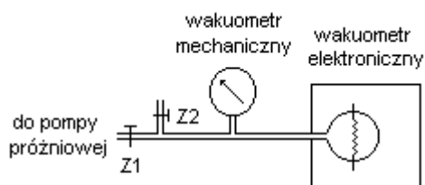
Rys.4. Układ skalowania próżniomierza elektronicznego
